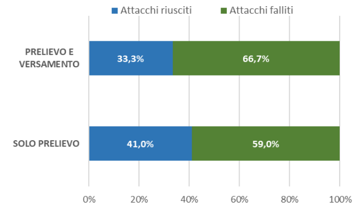
Attacchi 2024 per tipologia ATM ed esito
