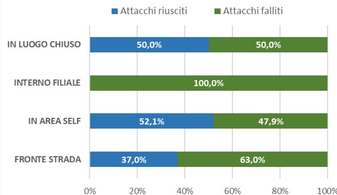
Attacchi 2024 per collocazione ATM ed esito
