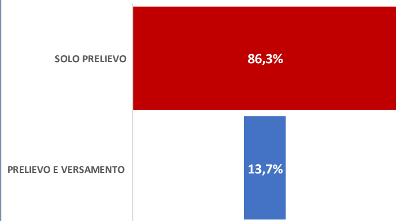
Attacchi ATM 2024 per tipologia dell'ATM
