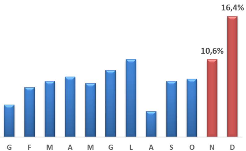
Attacchi per mese
