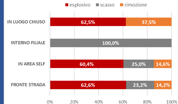
Attacchi 2024 per collocazione e modalità
