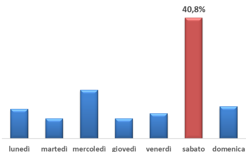
Attacchi per giorno della settimana
