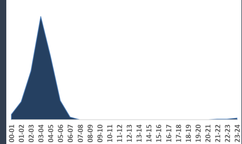
Attacchi per ora di accadimento
