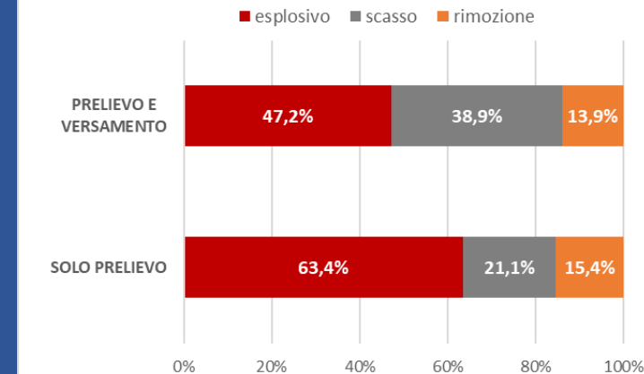
Attacchi 2024 per tipologia ATM e modalità
