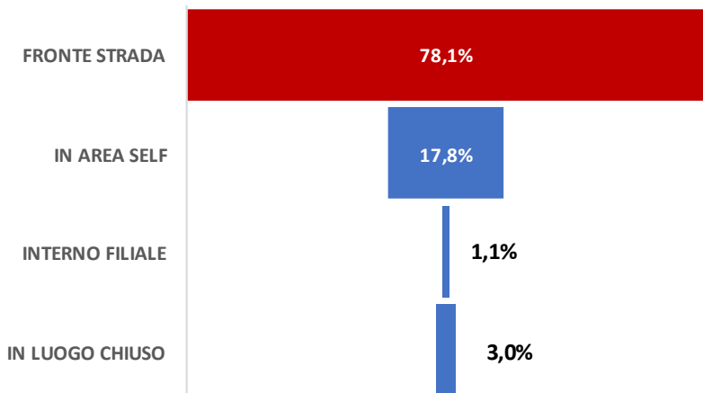
Attacchi ATM 2024 per collocazione dell'ATM
